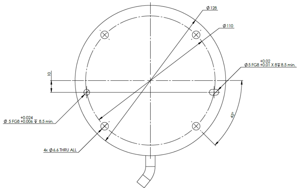
1.1: Undersidan av robotbasen
