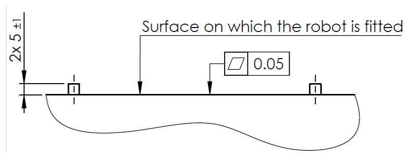
1.2: Monteringsplatta för robotbas
